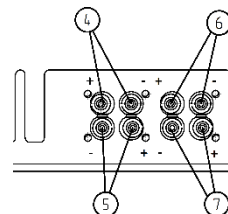
Rys. 6a Rozmieszczenie przetworników ciśnienia w wariantcie S2 / S4 / S
