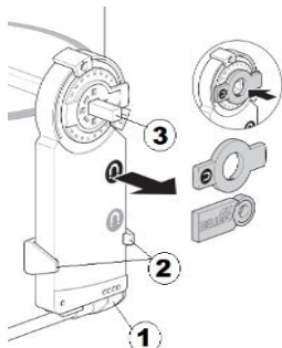
Rys. 31. Demontaż siłownika obejścia
