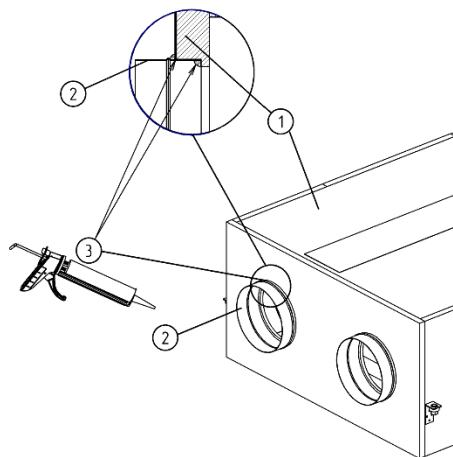
Rys. 21. Sposób wykonania izolacji przyłączy instalacji wentylacyjnych
