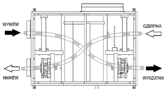
Rys. 8. Wykonanie podstawowe PRAWA (widok od góry)
