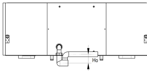
Rys. 20. Wymiarowanie H_o
