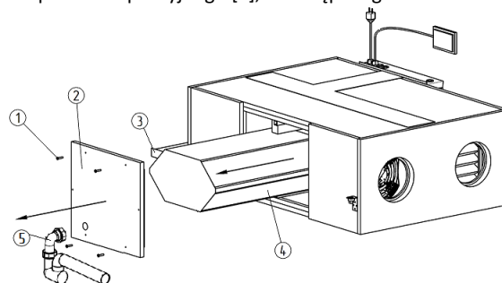
Rys. 29. Wymiennik odzysku ciepła UOC
