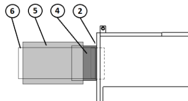
Rys. 22. Sposób wykonania izolacji przyłączy instalacji wentylacyjnych
