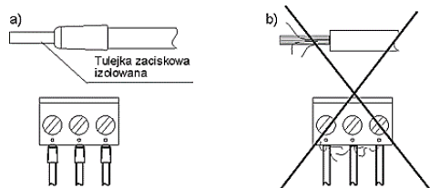
Rys. 23. Zabezpieczanie końców przewodów: a) -prawidłowe b) -nieprawidłowe
