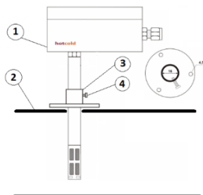
Rys. 25 Montaż czujników kanałowych
