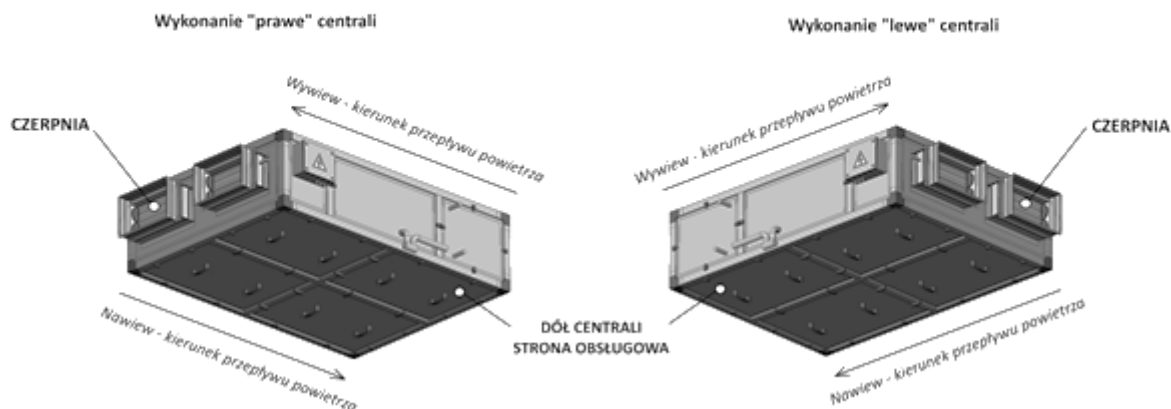
Rys. 7 Strona wykonania central podwieszanych (R-prawa, L-lewa)
