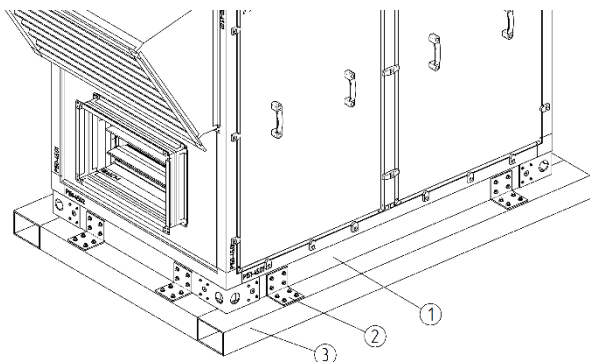
Rys. 9 Proponowany wariant zamocowania centrali do konstrukcji wsporczej
