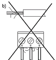
Rys. 21. Zabezpieczanie końców przewodów:
