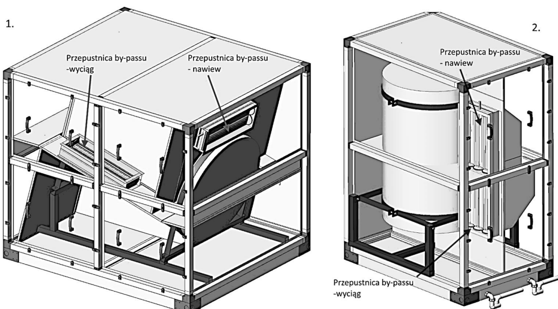
Rys. 25 Rozmieszczenie przepustnic by-pass (1-wariant WS-C; 2-wariant WS-G)
