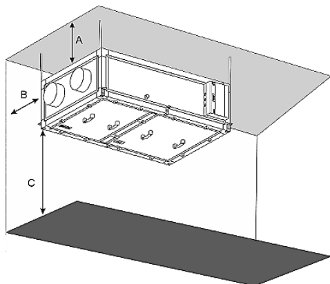
Rys. 12 Zalecana przestrzeń obsługowo-montażowa central podwieszanych
