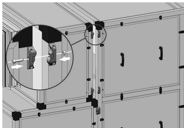
Rys. 13 Sposób łączenia pionowego modułów
