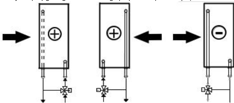
Rys. 20 Przykład przeciwpłdowego podłączenia nagrzewnicy i chłodziły wodnych
