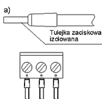
Rys. 21. Zabezpieczanie końców przewodów:
