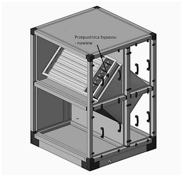
Rys. 28 Umieszczenie przepustnicy bypassu VEBAR-CS
