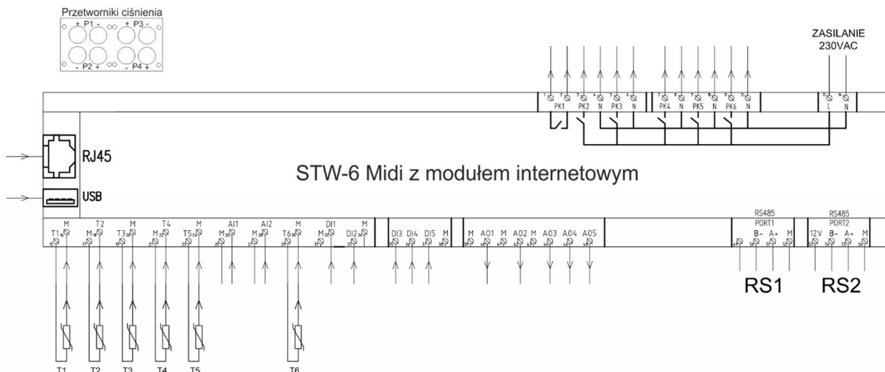
Schemat sterownika z wbudowanym modułem internetowym
