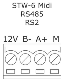
Rys. 36 Schemat podłączenia sterownika STW-6 midi do systemu BMS
