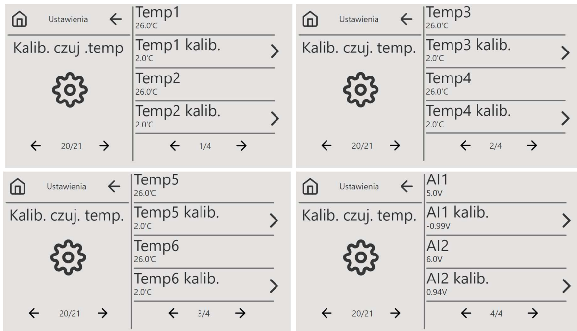
Rys. 43 Ekran kalibracji czujników
