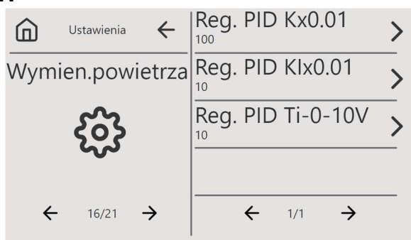
Rys. 39 Ekran ustawień wymiennika powietrza
