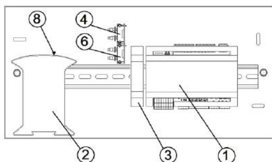
Rys. 7 Elementy szafy automatyki w wariacie S2/S4/S
