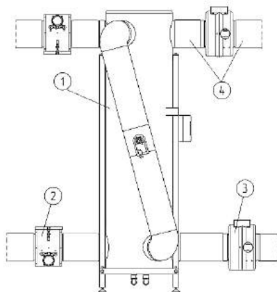
Rys. 28 Zestaw VENA z osprzętem w wariantcie kanałowym
