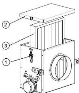
Rys. 38 Wymiana wkładu filtracyjnego
