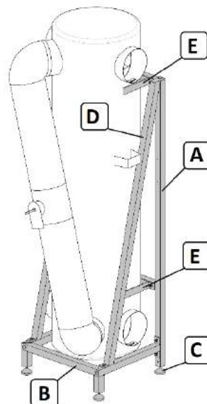
Rys. 20 Rama w wersji stojącej
