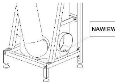
Rys. 12 Miejsce oznakowania przeznaczenia instalacyjnego króćca przyłączeniowego
