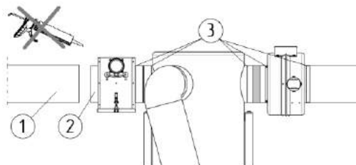
Rys. 31 Wykonanie przyłączy instalacji wentylacyjnej
