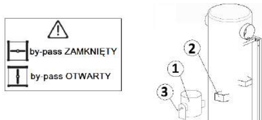
Rys. 26 Przepustnica obejścia UOC
