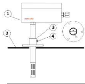
Rys. 36 Montaż czujników kanałowych
