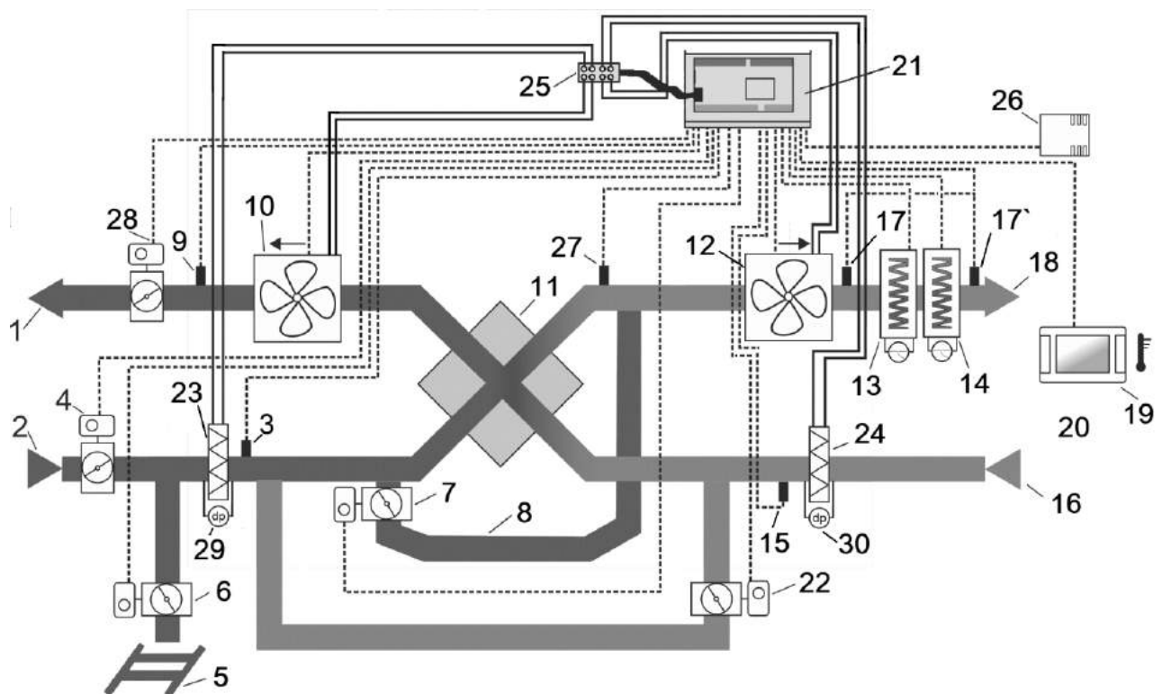
Rys. 16 Schemat ideowy centrali VENA Silver wersji XC
