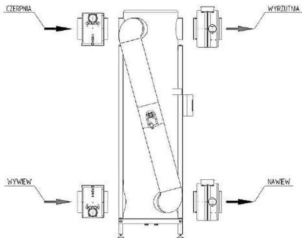
Rys. 10 Wykonanie PRAWA (podstawowe)
