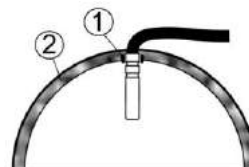
Rys. 35 Montaż czujnika temp. w kanale
