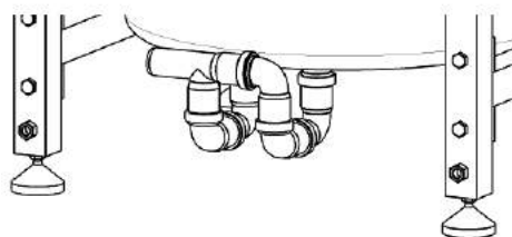
Rys. 23 Prawidłowe wykonanie syfonu zalewowego za pomocą kształtek
