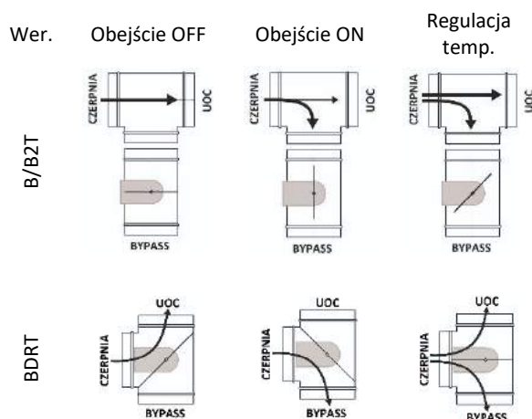
Rys. 27 Działanie przepustnic obejściowych
