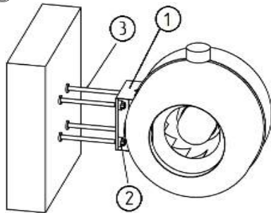
Rys. 30 Zalecany sposób montażu [1] i zaczep montażowy; [2] amortyzator gumowy; [3] pręt gwintowany
