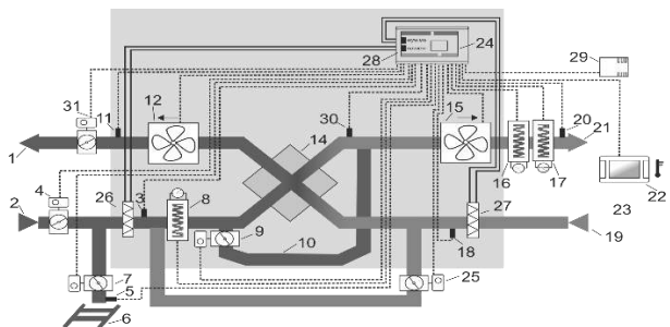
Rys. 17a Recyrkulacja z przepływem powietrza recyrkulowanego przez wymiennik ciepła
