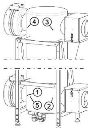
Rys. 13 Rozmieszczenie czujników temp. strona wykonania PRAWA (widok od „pleców”)
