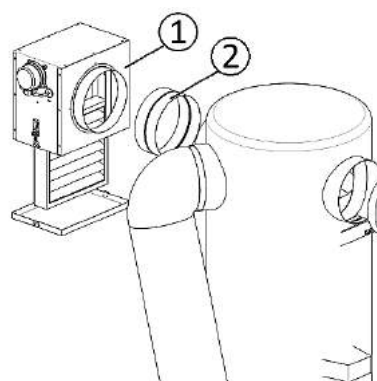
Rys. 29 Montaż skrzynek filtracyjnych bezpośrednio na króćcach wymiennika
