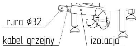
Rys. 24 Prawidłowo wykonana izolacja termiczna
