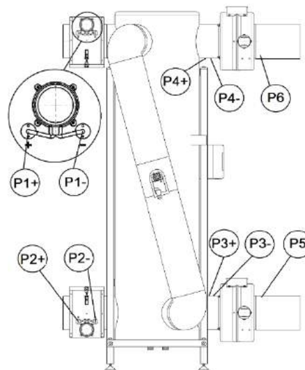
Rys. 15 Miejsca pomiaru ciśnienia wykonanie PRAWO (wariant S2)
