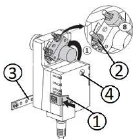
Rys. 28 Sposób odblokowania i montażu siłownika obejścia
