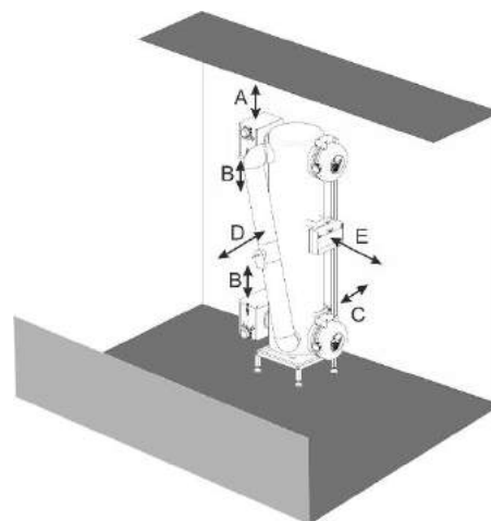
Rys. 18 Wymagane min. odległości serwisowe
