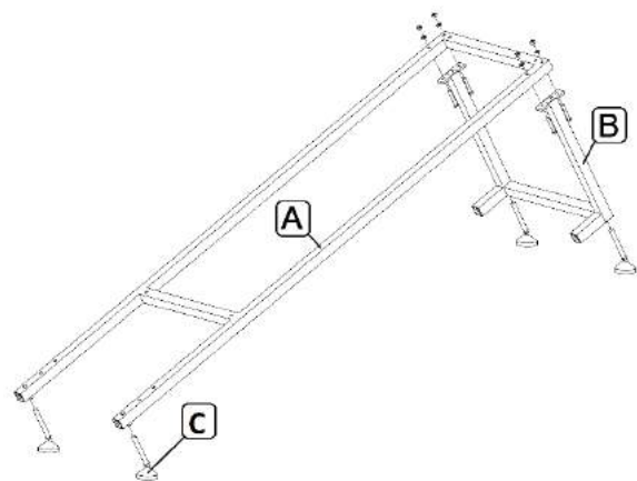
Rys. 21 Leżąca pozycja pracy – rama standardowa
