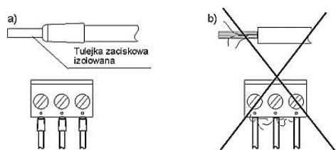
Rys. 33 Zabezpieczanie końców przewodów: a) prawidłowe, b) nieprawidłowe
