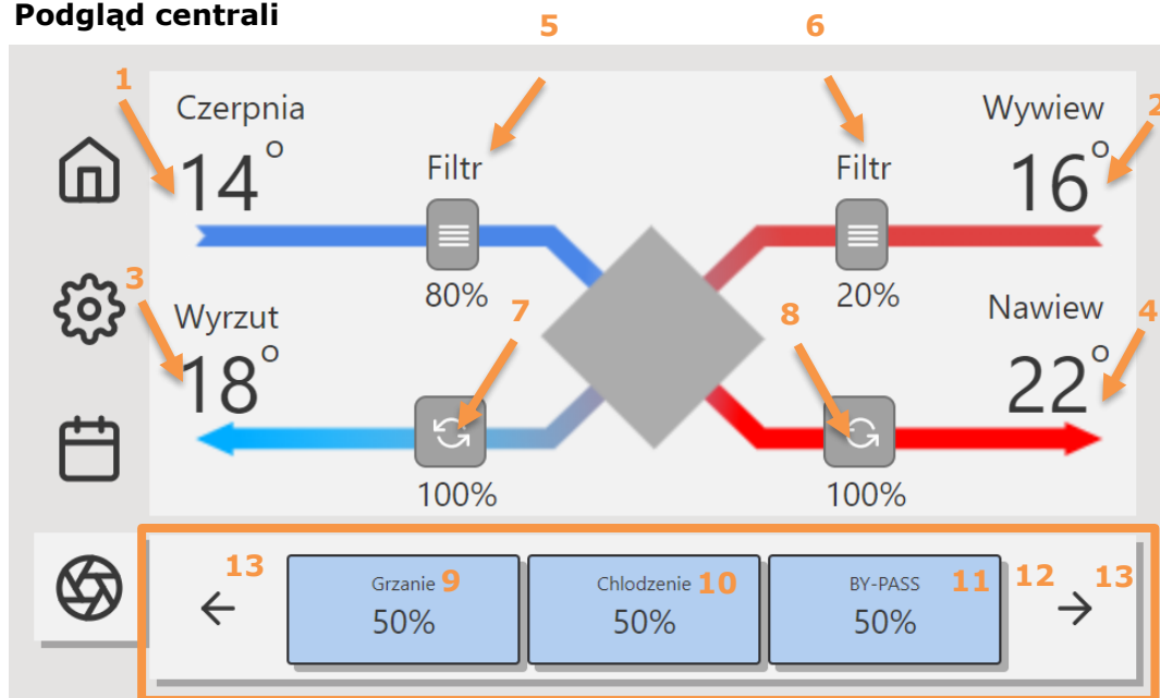
Rys. 2 Okno podglądu centrali
