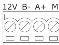
Rys. 36 Schemat podłączenia sterownika STW-6 midi do systemu BMS
