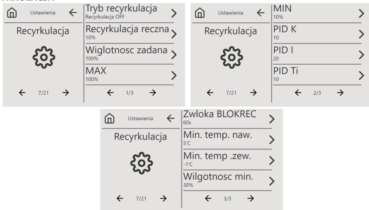
Rys. 34 Ekrany ustawień parametrów recyrkulacji
