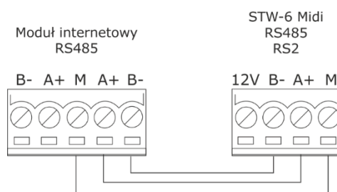
Rys.19 Schemat połączeniowy modułu ze sterownikiem STW-6 Midi
