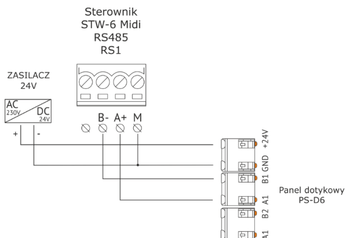
Rys. 17 Podłączenie PS-D6 ze sterownikiem, przy odległości większej jak 30m.
