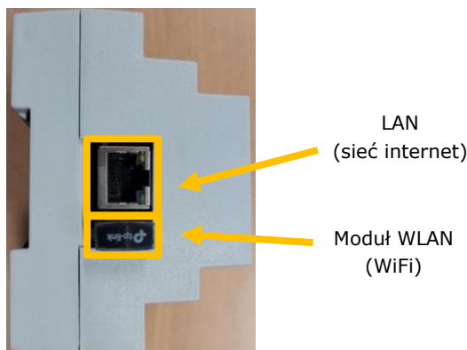
Rys. 20 Podłączenie modułu internetowego wbudowanego
