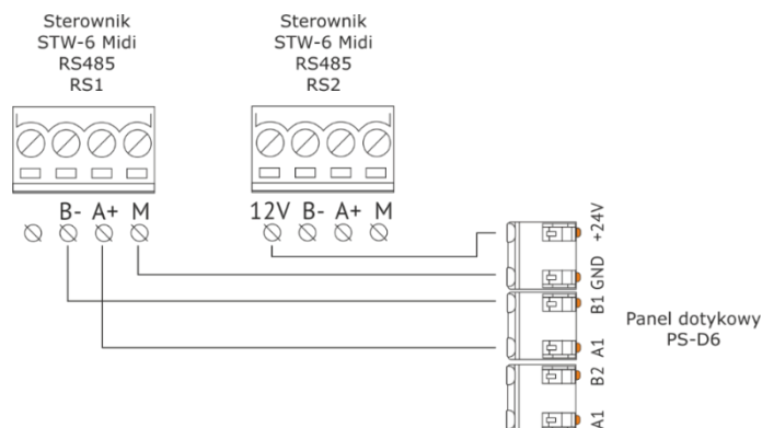
Rys. 16 Podłączenie PS-D6 ze sterownikiem, długość przewodu do 30m
