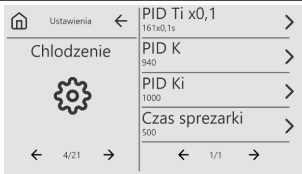
Rys. 27 Ekran ustawień parametrów chłodzenia
