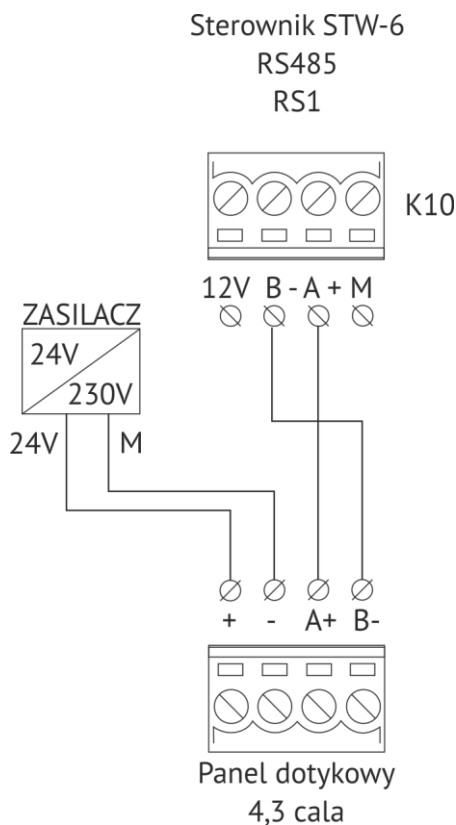
Rys. 1 Schemat podłączeniowy
